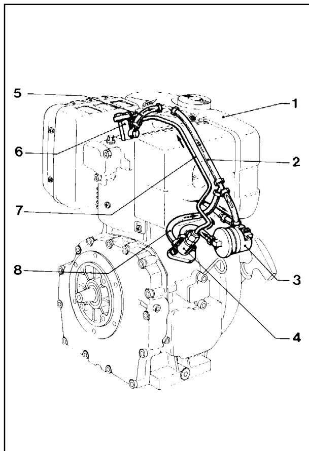
Circuito de alimentación/inyección para 15 LD 315-350-400-440
