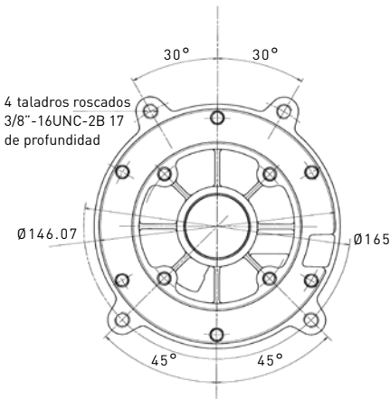
Acoplamiento SAE J609
