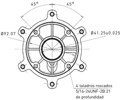
Tipo de acoplamiento B - 15 LD350-350S
