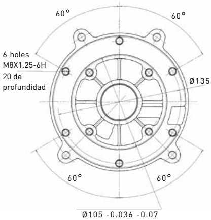
Tipo de acoplamiento A - 15 LD225-225S
